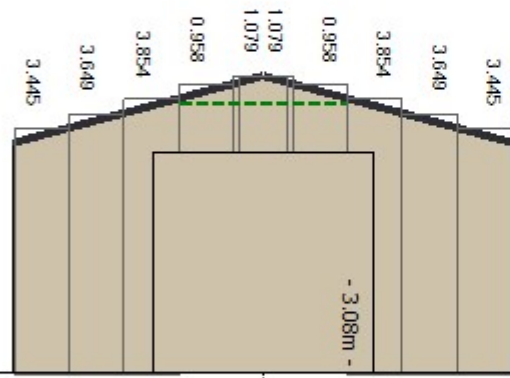
Left End
